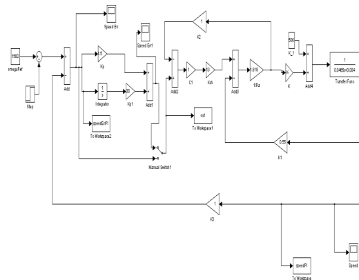
P-I CONTROLLER
