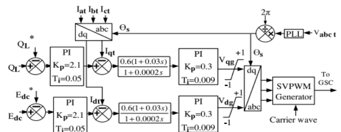
Fig. 3. GSC controller.
