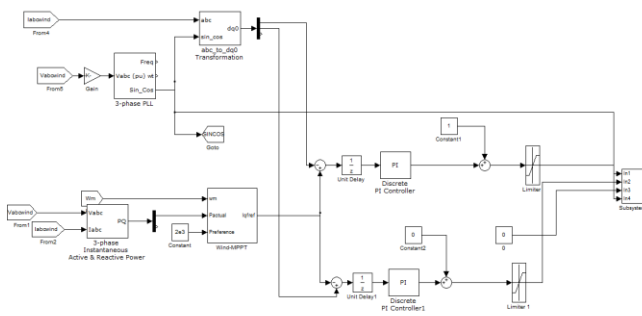
Fig 10. PMSG controller
