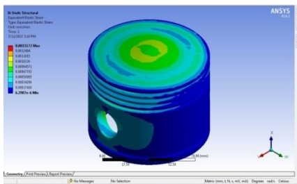
Al 6061+b4c
