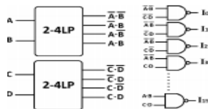
Fig:4-16LPI line decoder
