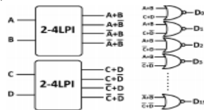
Fig:4-16LP line decoder
