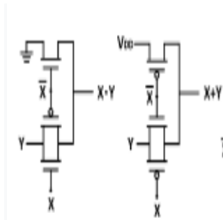
Fig: AND/OR gates using TGL
