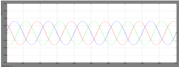
(d) Simulation waveform of load voltage VabcL
