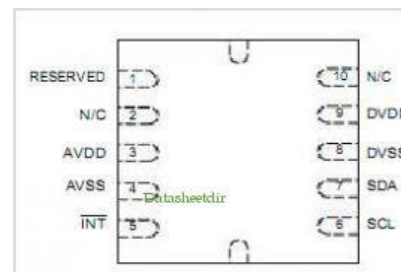
Fig.6. MEMS IC
