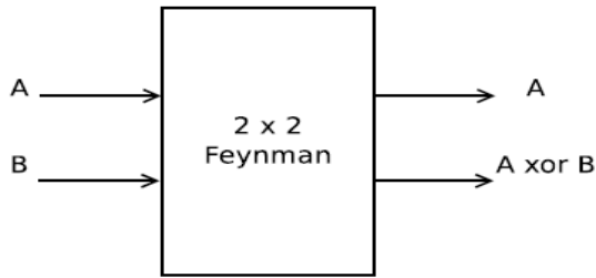
Fig. 4: Feynman Gate
