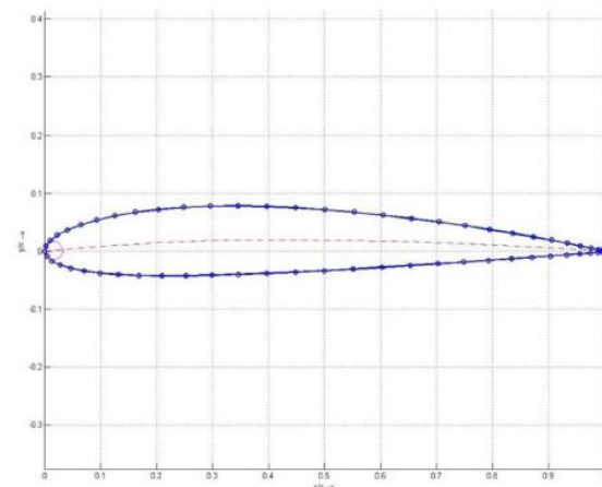
Fig. 1: NACA 2412 Aero foil Design
