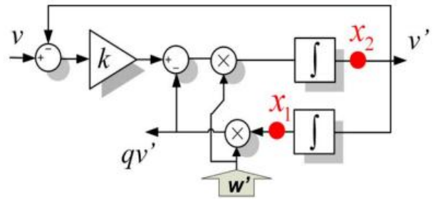
SOGI - QSG
