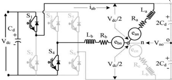
Fig. 5. VSI feeding a BLDC motor.
