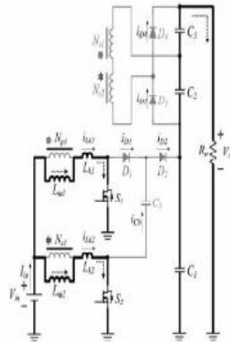
(d) Mode-4 [t3, t4].
