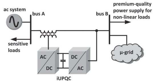
Fig1 : simulation circuit
