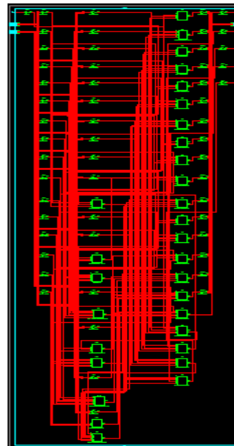
Fig3. TTL of 16bit CSA
