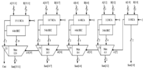
Fig1. Modified 16 Bit CSA
