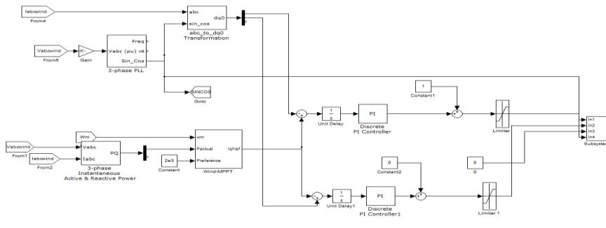
Fig 10. PMSG controller
