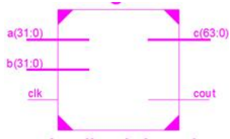
Fig. 3 R.T.L Schematic
