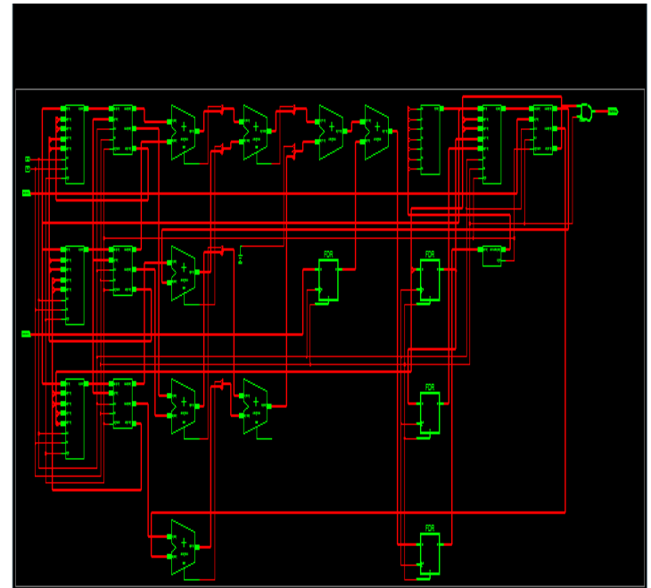
Fig: RTL Schematic
