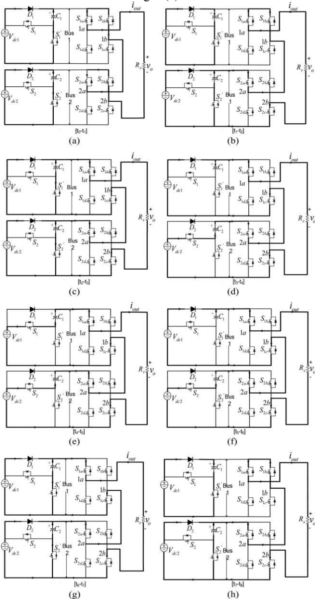
Fig.4. Active circuits for different operation intervals in the operational mode 1: (a) t0 - t1 ; (b) t1 - t2 ; (c) t2 - t3 ; (d) t3 - t4 ; (e) t4 - t5 ; (f) t5 - t6 ; (g) t6 - t7 ; (h) t7 - t8 .
